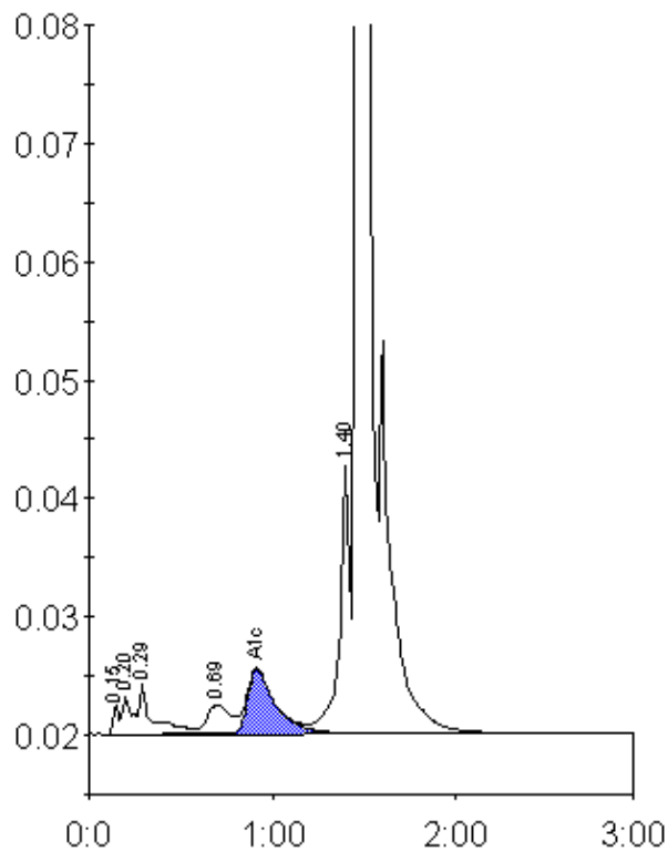
Peak table - ID: 10572015
